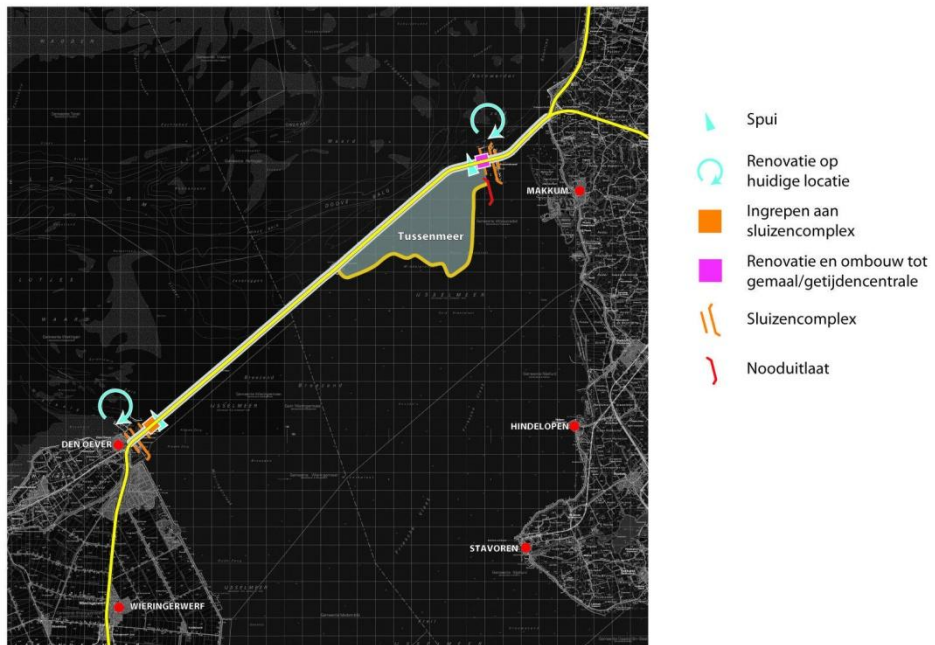
Figuur 4.14 WaterMachine zonder ESA (WMz)
