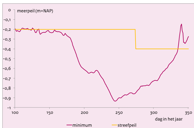
Figuur 6.5 Minimum IJsselmeerpeil in 2100 in het W+scenario*
