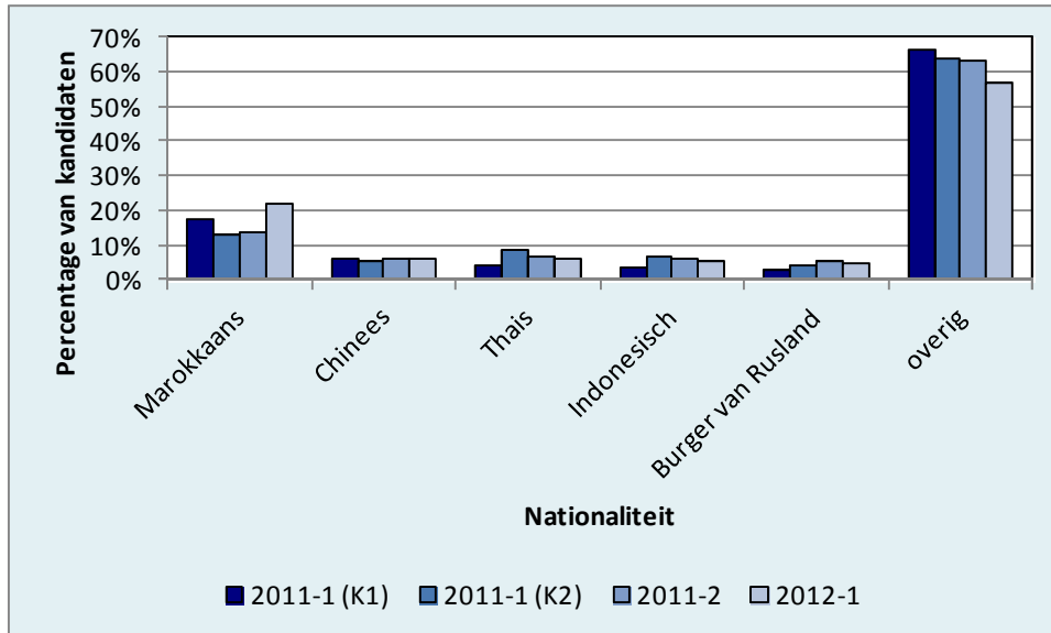
Figuur 10: Resultaten van het eerste basisexamen inburgering naar nationaliteit sinds 2011
