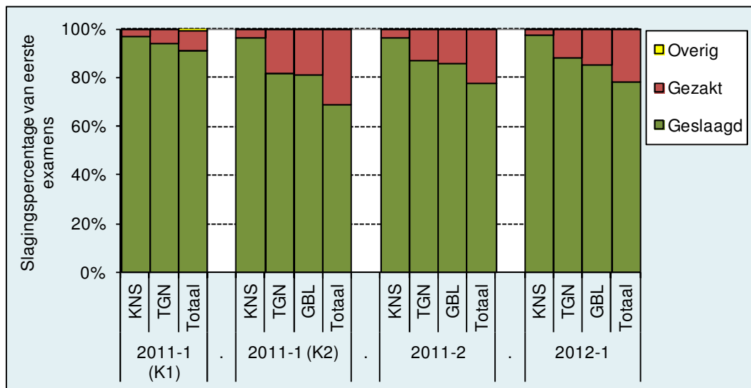
Figuur 4: Resultaten van het eerste basisexamen inburgering vanaf 2011
