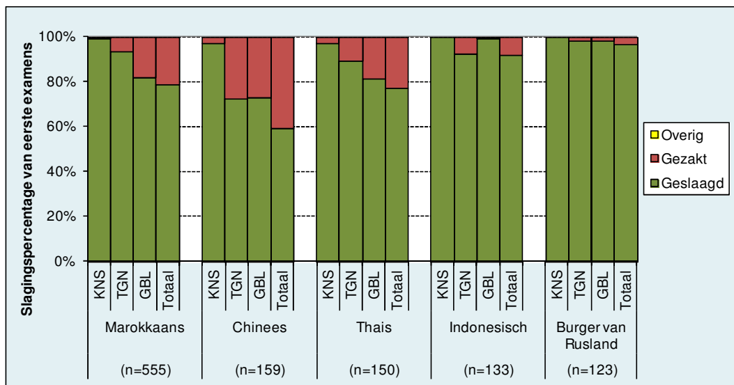
Figuur 11: Resultaten van het eerste basisexamen inburgering naar nationaliteit in 2012-1
