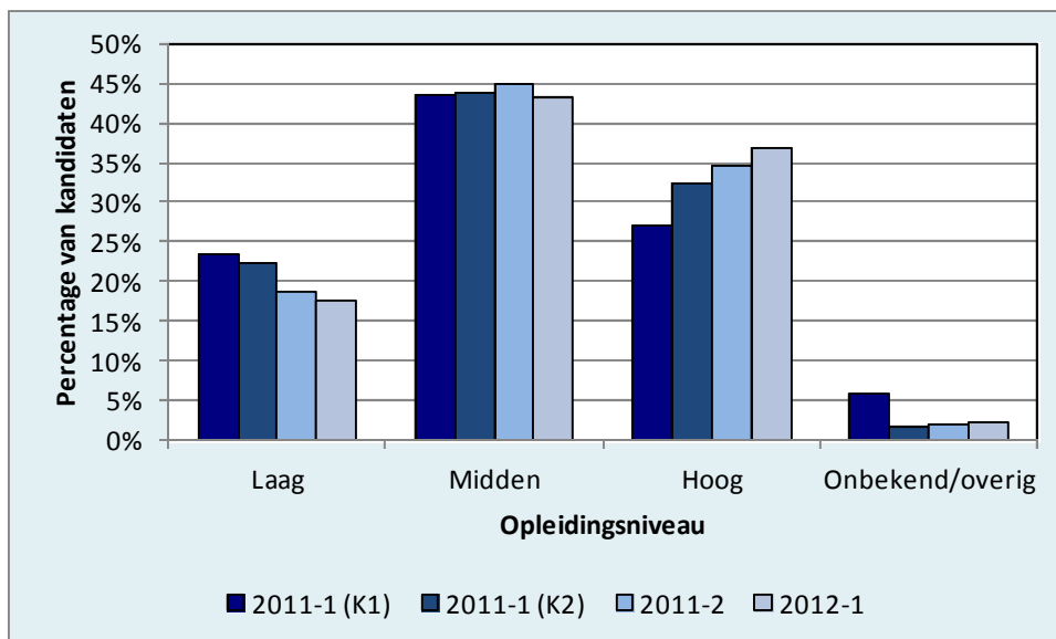
Figuur 8: Aandelen per opleidingsniveau sinds 2011 15
