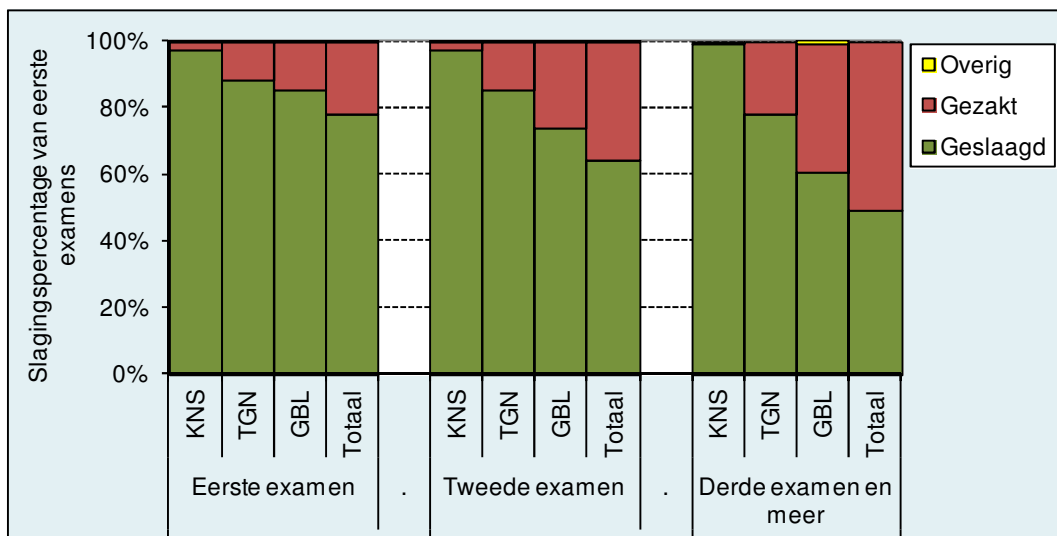
Figuur 5: Resultaten van het eerste basisexamen inburgering naar aantal examens in 2012-1
