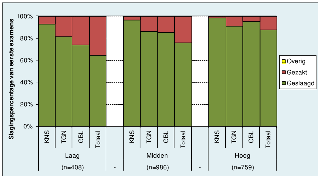
Figuur 9: Resultaten van het eerste basisexamen inburgering naar opleidingsniveau in 2012-1
