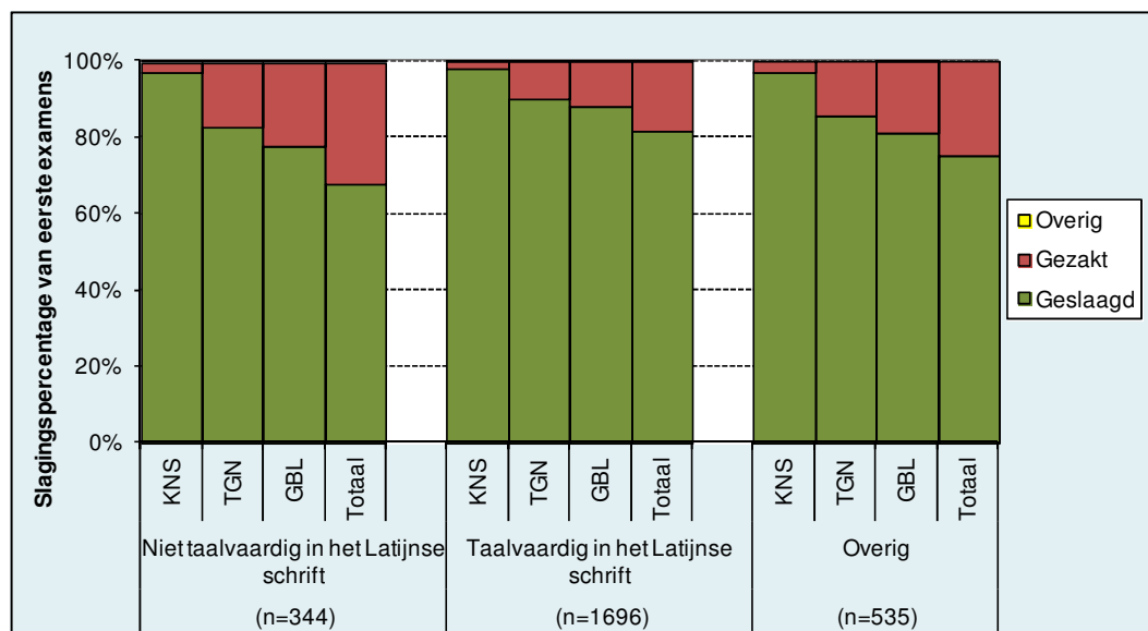
Figuur 12: Resultaten van het eerste basisexamen inburgering naar gealfabetiseerdheid in het Latijnse schrift in 2012-1
