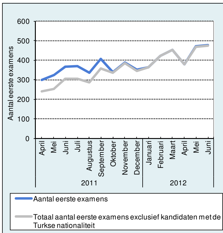
Figuur 15: Aantal eerste examens per maand vanaf april 2011: inclusief en exclusief kandidaten met de Turkse nationaliteit
