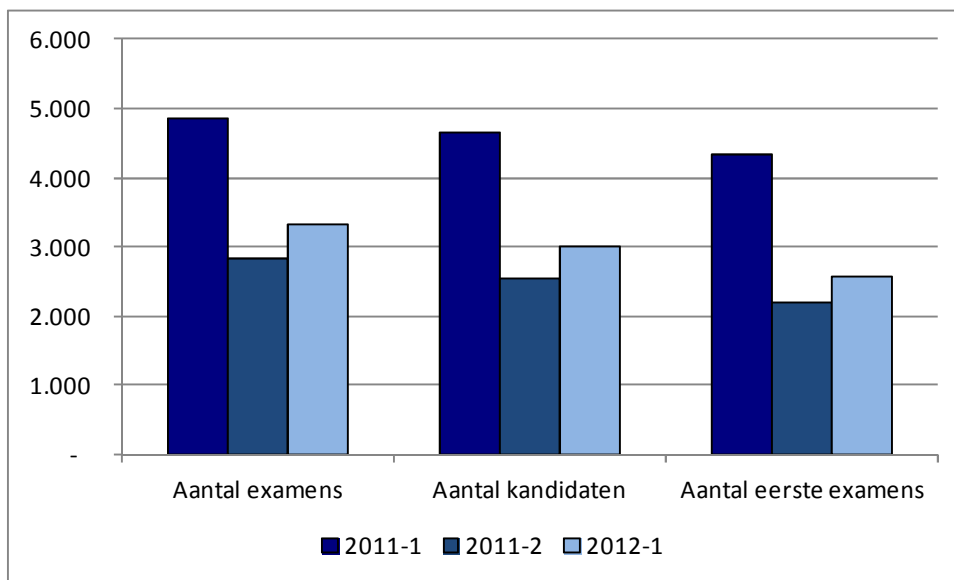
Figuur 3: Aantal examens, aantal kandidaten en aantal eerste examens
