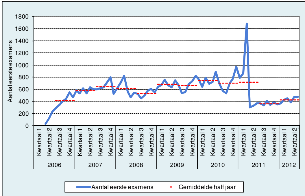
Figuur 14: Aantal eerste examens per maand vanaf 2006
