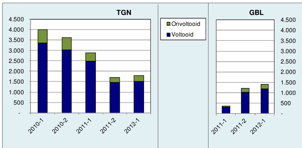
Figuur 2: Aantal en status van oefenexamens sinds 2010 (Bron: Ordinate en CINOP)
