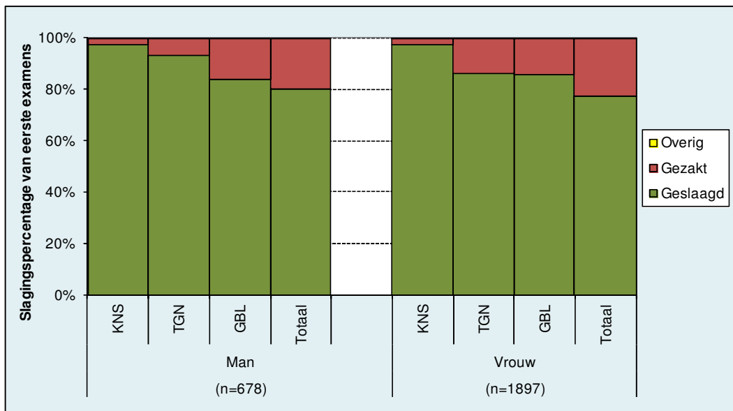
Figuur 6: Resultaten van het eerste basisexamen inburgering naar geslacht in 2012-1
