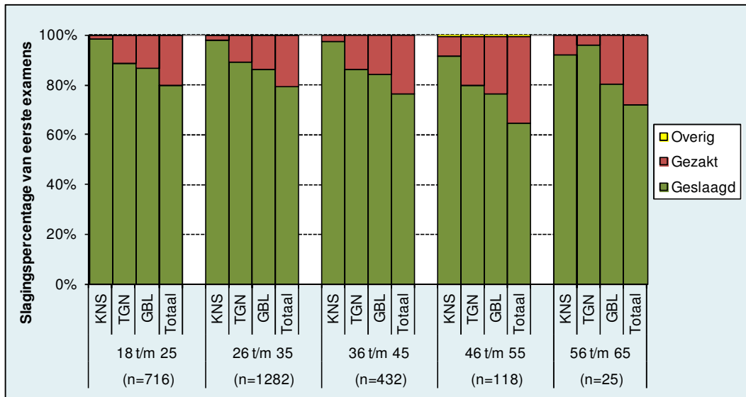
Figuur 7: Resultaten van het eerste basisexamen inburgering naar leeftijd in 2012-1
