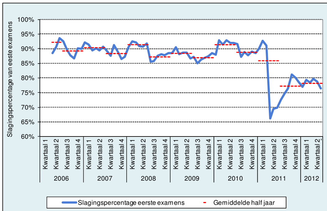
Figuur 13: Slagingspercentage van eerste examens per maand vanaf 2006
