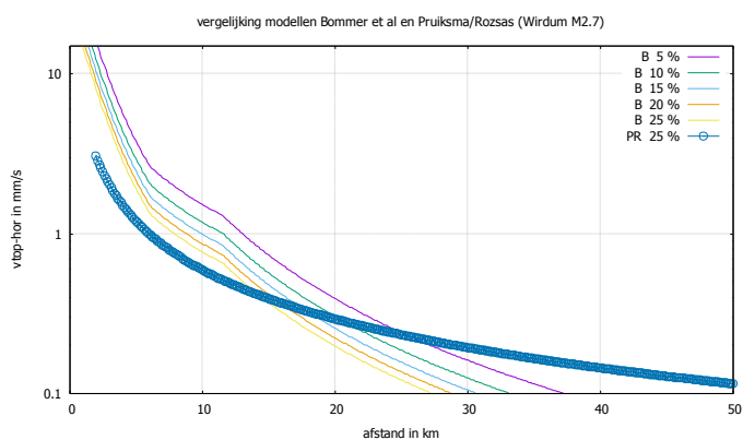
Figuur 7.5: vergelijking van de modellen van Bommer et al (aangeduid met B) en Pruiksm/Rozsas (aangeduid met PR) voor de beving Wirdum (2015-01-06) met magnitude 2,7.
