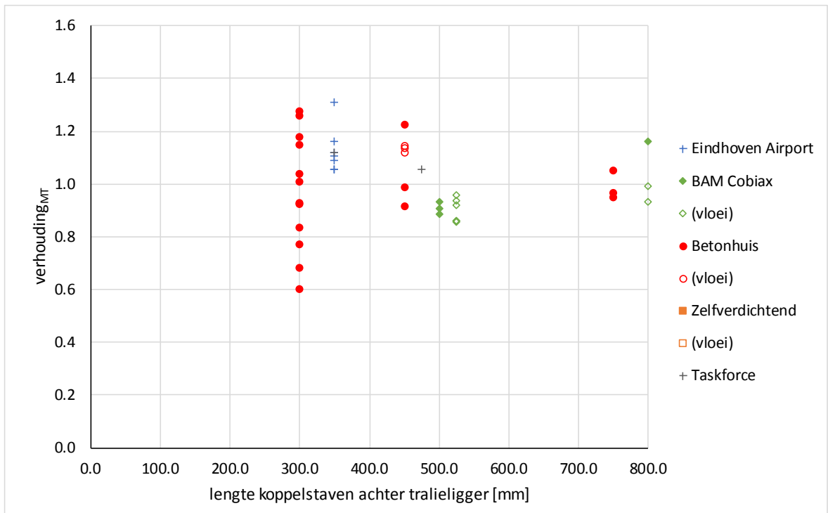
figuur D-3 Relatie lengte koppelwapening achter de tralieligger en verhouding MT
