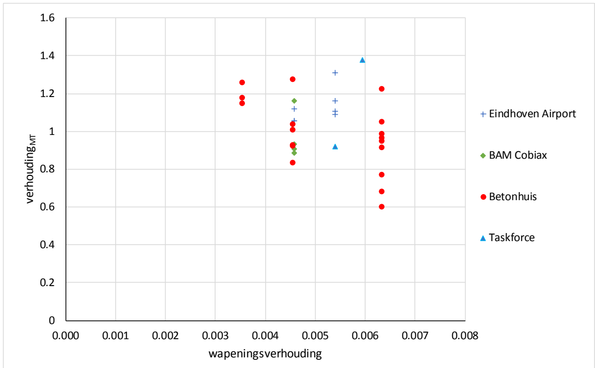
figuur D-5 Relatie wapeningsverhouding koppelwapening en verhouding _{MT}
