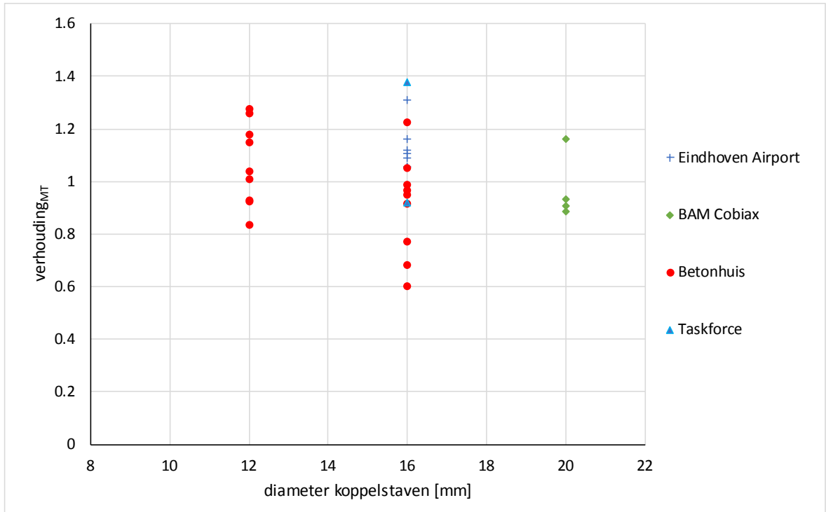
figuur D-4 Relatie diameter koppelwapening en verhouding _{MT}
