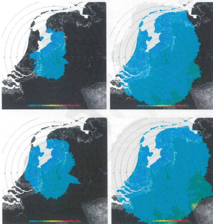
Figuur 4: Line-of-sight diagrammen voor de huidige antennehoogte (boven) en een antennehoogte van 60 m boven het maaiveld (onder). Links: doelhoogte 1000 voet, rechts: doelhoogte 5000 voet. De afstanden bij de ringen zijn in NM.
