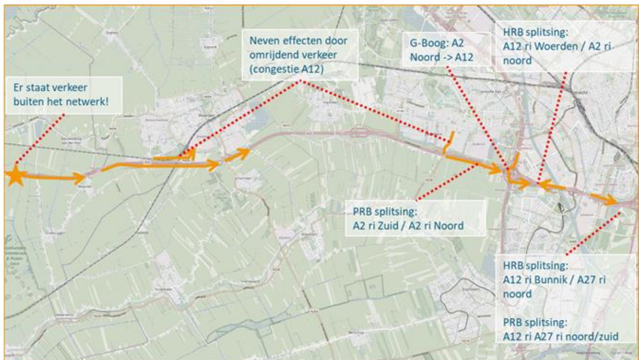
Figuur 13: Knelpunten regio Oost 2030 ochtendspits
