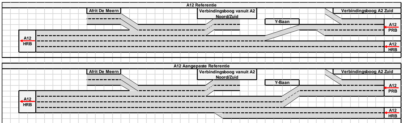
Figuur 12: Schematische weergave maatregelen op Y-Baan in knooppunt Oudenrijn, vergelijking tussen Referentie (boven) en aangepaste Referentie (onder)
