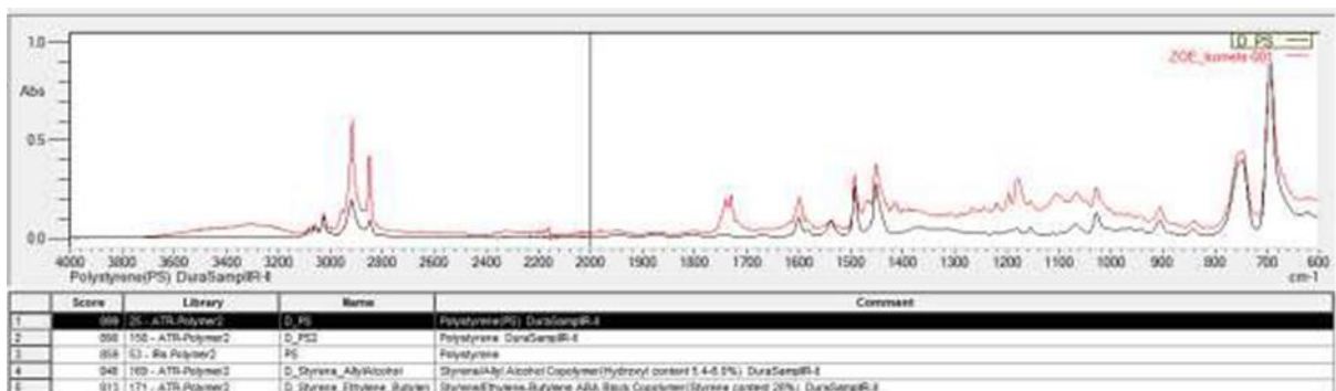
Figuur 6. Spectrum van polystyreen (PS) uit de FTIR bibliotheek (zwart) en het gecombineerd spectrum van de door de Zoe verloren PS-korrels (rood).
