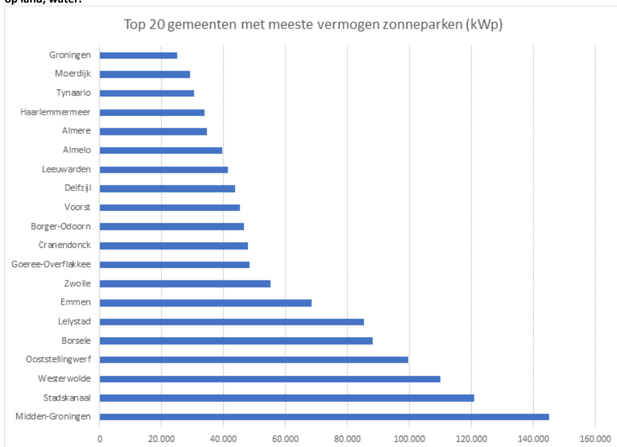
Figuur 3.3 – Opgesteld vermogen zonneparken per gemeente (20 gemeenten met het meeste vermogen), in kWp op land, water.
