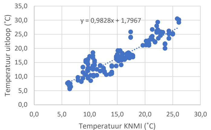
Figuur 18 Relatie tussen de temperatuur boven de vloer van de uitloop en de KNMI temperatuur van het dichtstbijzijnde weerstation ( ^{\circ}C )
