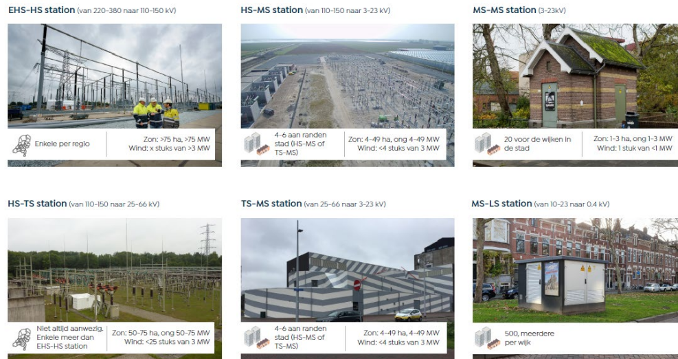
Afbeelding 2.2 Typen elektriciteitsstations
