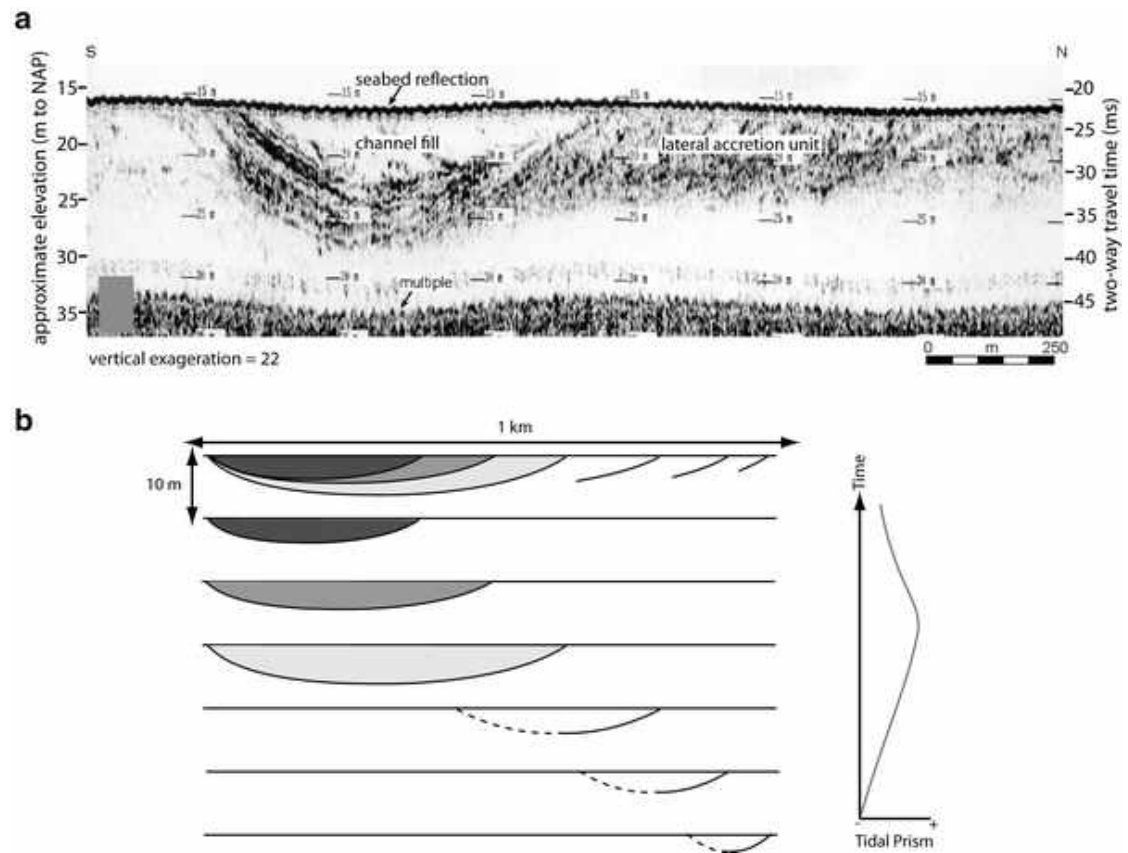
Figuur 3.4 Voorbeeld van geofysische waarneming van oude verlande geulstructuren onder een zeebodem
