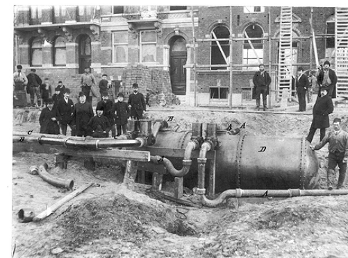
DISTRICT RESERVOIR XXXX IN DE ROEMER VISSCHERSTRAAT. A. WAFERBUIDEN. B. CENTRALE LUCHTBUS. C. CENTRALE TRANSPORTBUS. D. RESERVOIR RINGELN. DIA. 12976.
