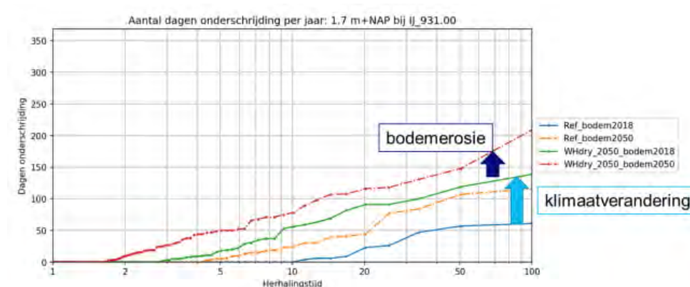
Figuur G2 Kans op en duur van overschrijding van het kritieke peil voor waterinlaat naar de Twentekanalen in de huidige situatie, en in 2050 bij veranderd klimaat en bij veranderde rivierbodempligging
