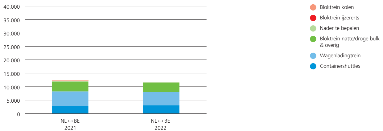
Grafiek 4.6: Ontwikkeling # goederentreinen per treinsoort op de grens Nederland – België in 2021 en 2022
