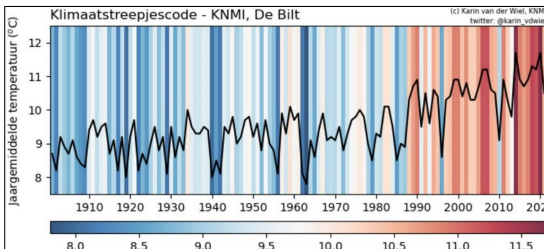
Figuur 7.1.1 De KNMI Klimaatstreepjescode bijgewerkt tot en met 2021. Blauwe streepjes tonen relatief koude jaren, rode relatief warme jaren. Bron: KNMI 2022
