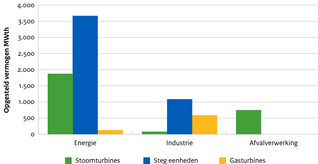
Figuur 2.6 Grote warmtekrachtkoppeling (WKK) installaties (>20 MWe) in 2022.
