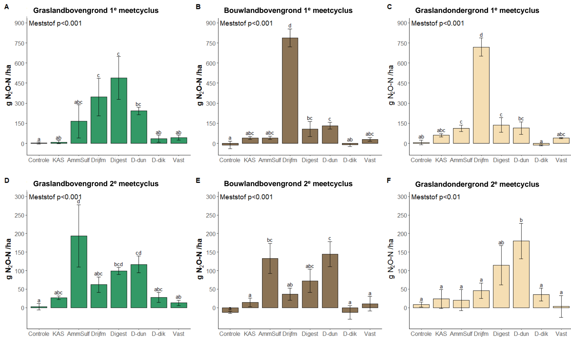
Figuur 3.1 Cumulatieve N 2 O-emissies gemeten over 40 dagen in de 1 e cyclus en 27 dagen in de 2 e cyclus voor de drie bodemsoorten; graslandbovengrond, bouwlandbovengrond en graslandondergrond. Foutenbalken geven de standaardfout weer (n=4 voor Controle, AmmSulf, Digest, D-dun, D-dik, Vast; n=6 voor KAS, Drijfm). Balken met dezelfde letters zijn niet significant verschillend (p<0.05). N.B. Let op de verschillen in schaal voor de Y-assen voor de eerste en tweede meetperiode.
