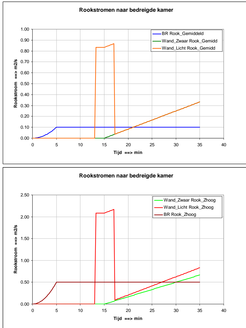
Figuur E.1a+b: Modellering van de gemiddelde waarden (figuur a) en zeer hoge waarden (figuur b) voor de rookstromen naar de bedreigde kamer vanuit de brandruimte (BR) en vanuit de constructie (voor thermisch lichte en zware beplating). Deze rookstromen dienen als invoer voor de berekening van de rookdichtheden in de bedreigde ruimten.
