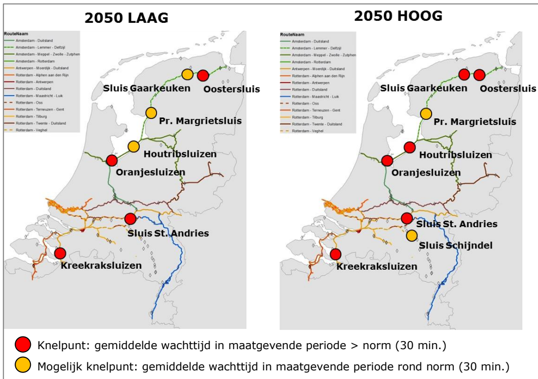
Figuur 12: Knelpuntenbeeld sluiscapaciteit 2050 (scenario's Laag en Hoog)
