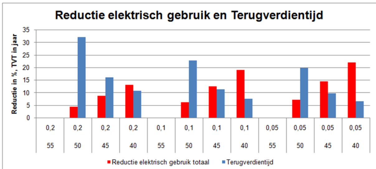
Figuur 6. Reductie energiegebruik en terugverdiertijd combiwarmtepomp met booster voor een eengezinswoning met gebruiksoppervlakte van 100 m 2 .
