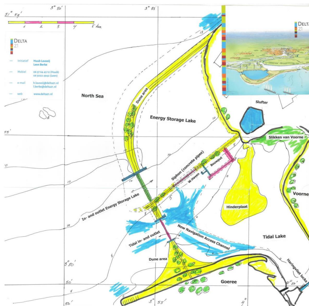
Figuur 6 Ontwerp van het Delta21-concept (Delta21, 2020)
