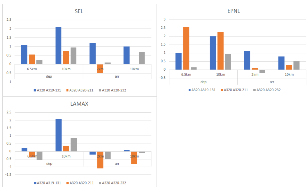
Figuur 26: Verschil in SEL, EPNL en LAMax voor de Airbus A320 familie na toepassen geluidcorrectie.
