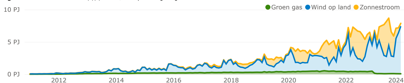
Figuur 11.1 Productie binnen SDE(+)(+) van zon, wind op land en groen gas
