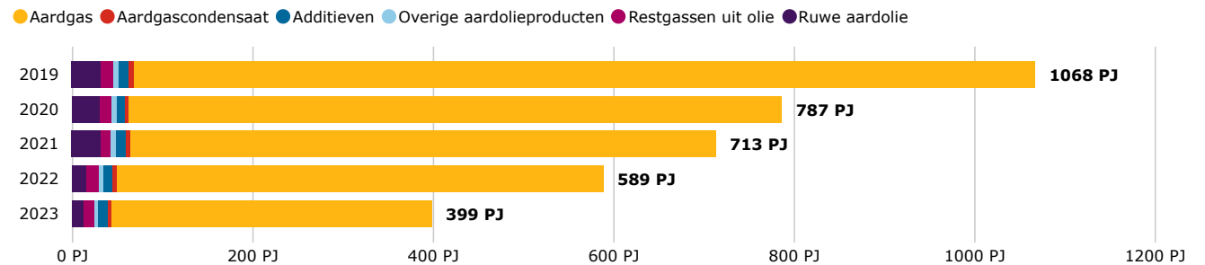
Figuur 5.1 Winning van fossiele koolstofdragers in Nederland
