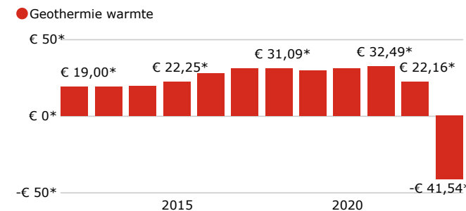
Figuur 11.4 Onrendabele top van geothermie
