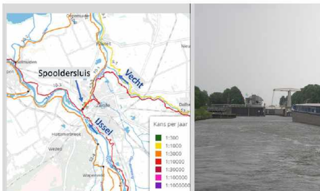
Figuur 2-1 Ligging en foto van de Spoldersluis.
